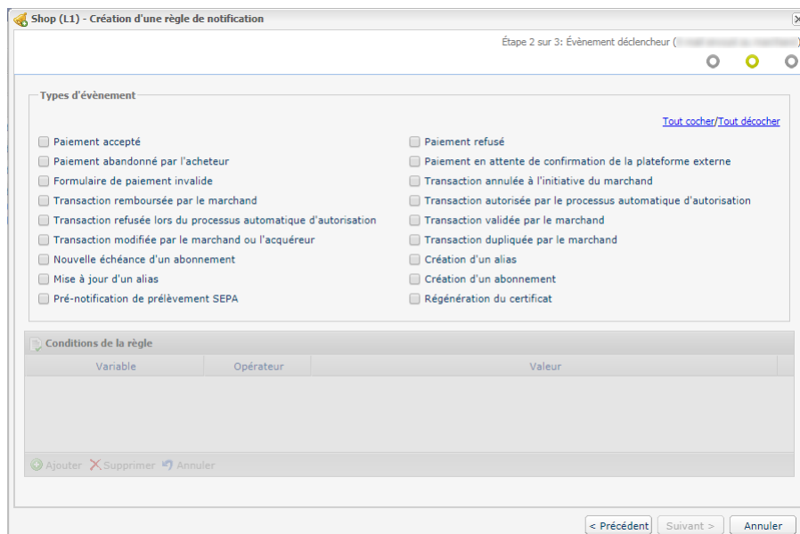
Image 2 : Assistant de création d'une règle de notification - Étape 2
